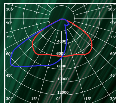
ASYMMETRINEN, AREA VALONJAKO (VAIN SKL20)
