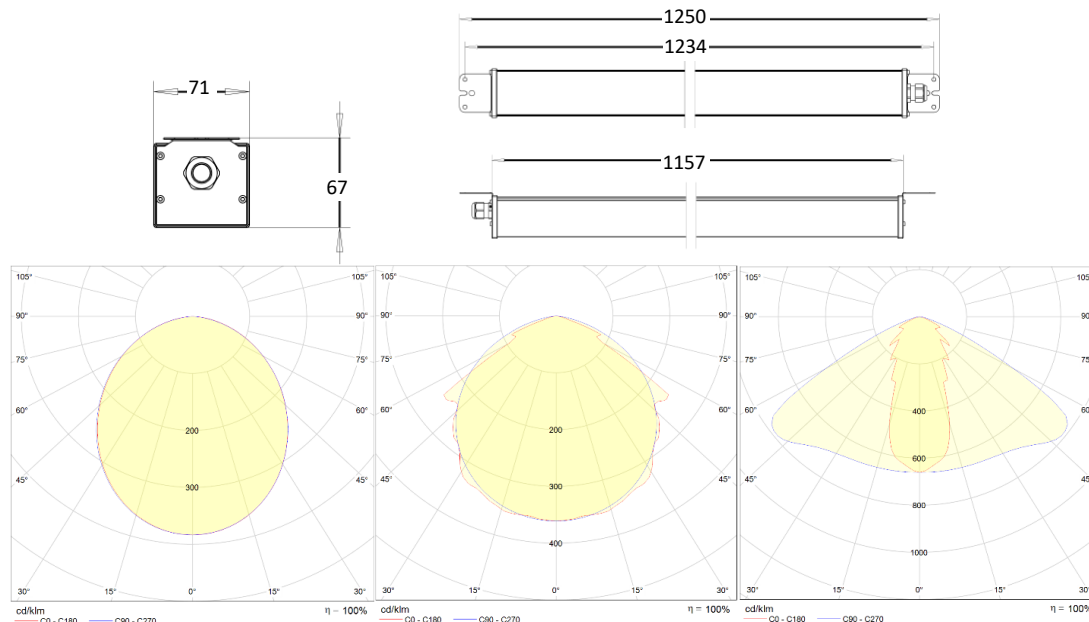
Opaalikuvun valonjako
