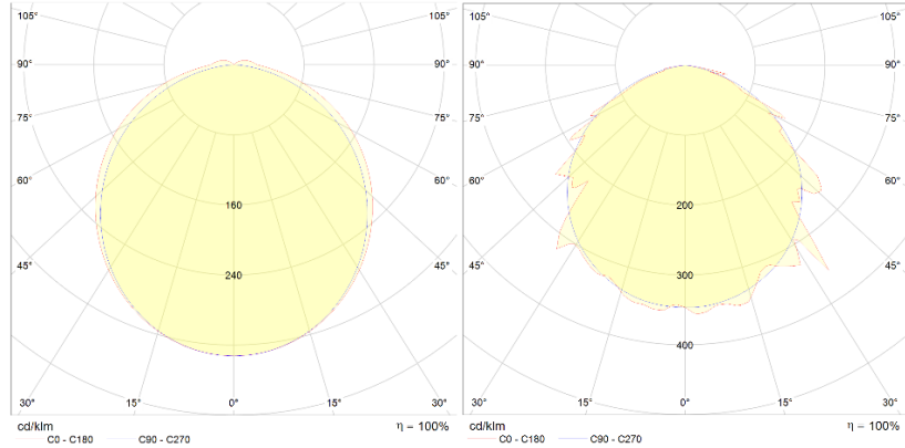
Opaalikuvun valonjako
