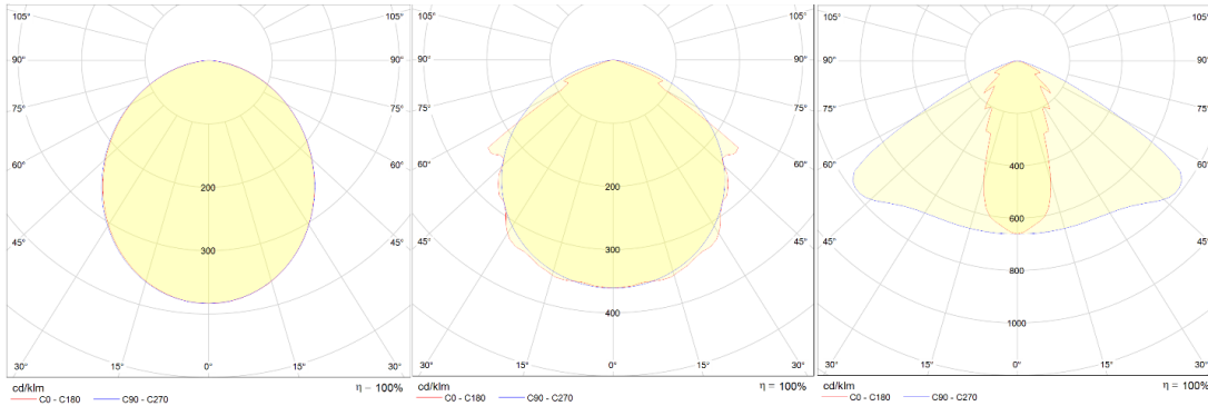
Opal kuvun valonjako
