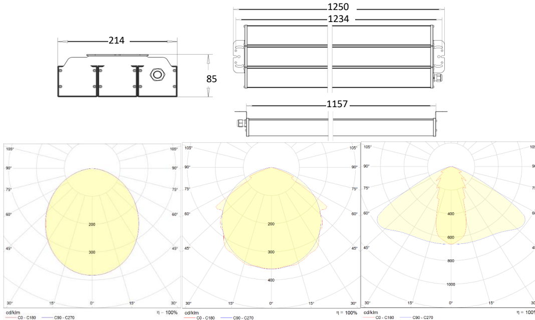
Opaalikuvun valonjako Kirkkaan kuvun valonjako Linssivalaisimen valonjako
