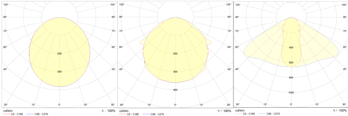
Opaalikuvun valonjako
