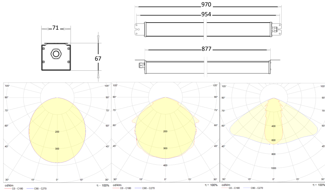
Opaalikuvun valonjako
