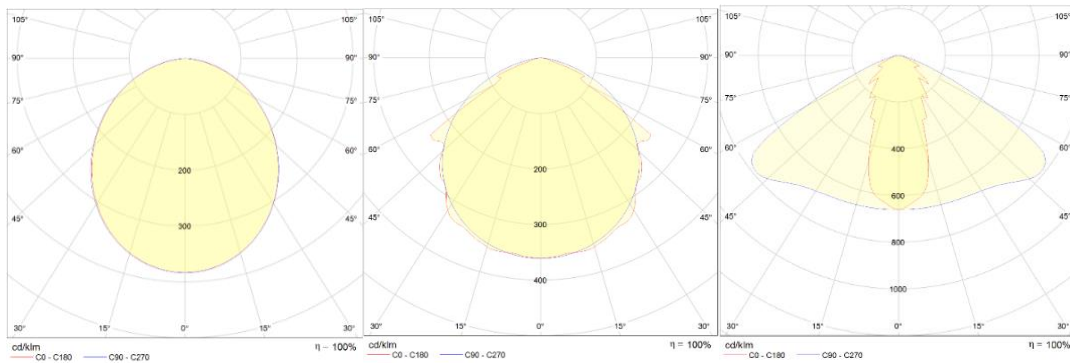
Opaalikuvun valonjako
