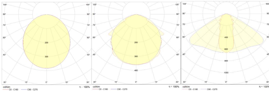
Opaalikuvun valonjako
