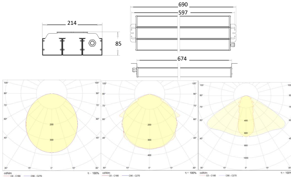
Opaalikuvun valonjako Kirkkaan kuvun valonjako Linssivalaisimen valonjako
