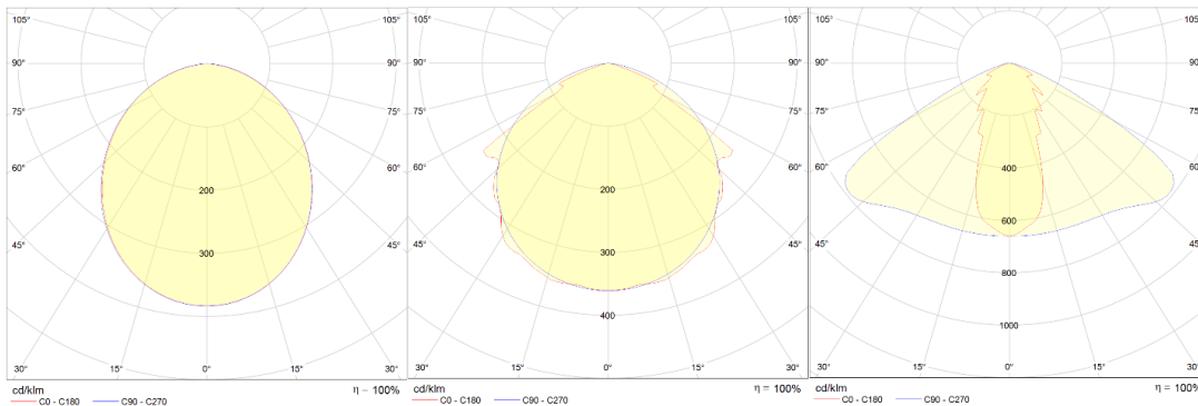
Opaalikuvun valonjako
