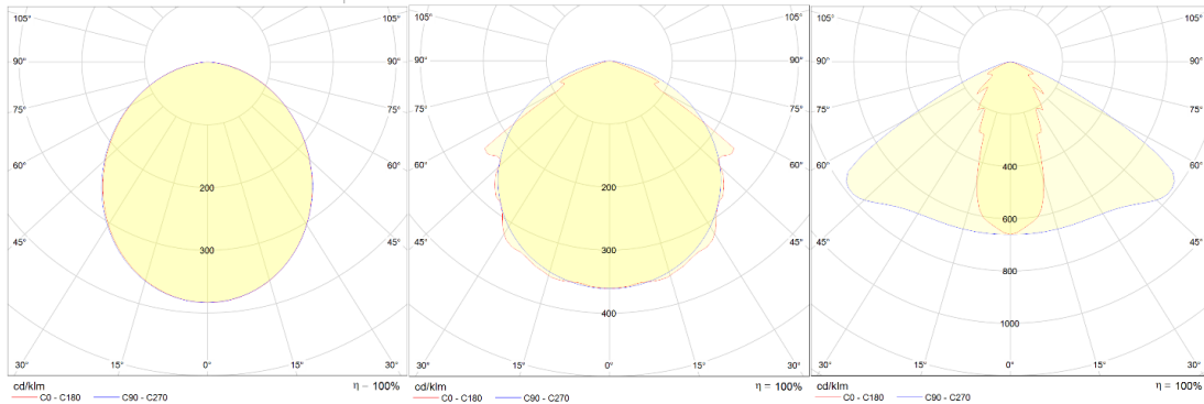
Opaalikuvun valonjako
