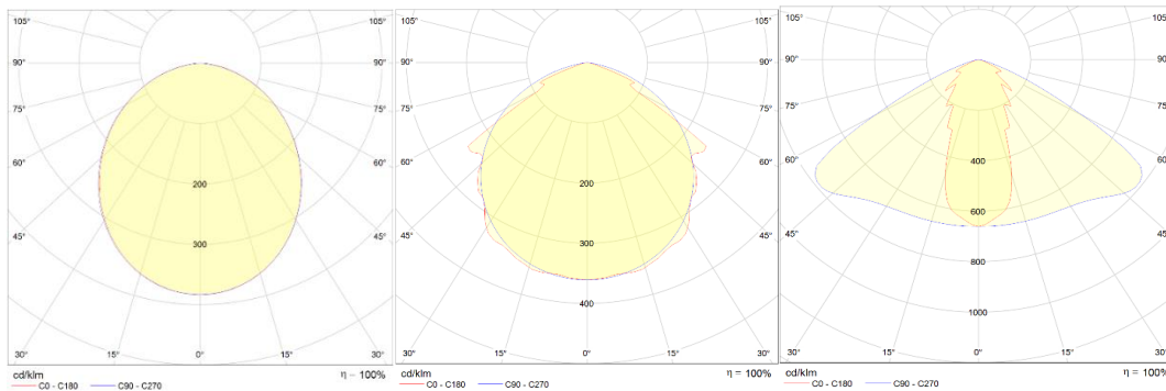
Opaalikuvun valonjako Kirkkaan kuvun valonjako Linssivalaisimen valonjako
