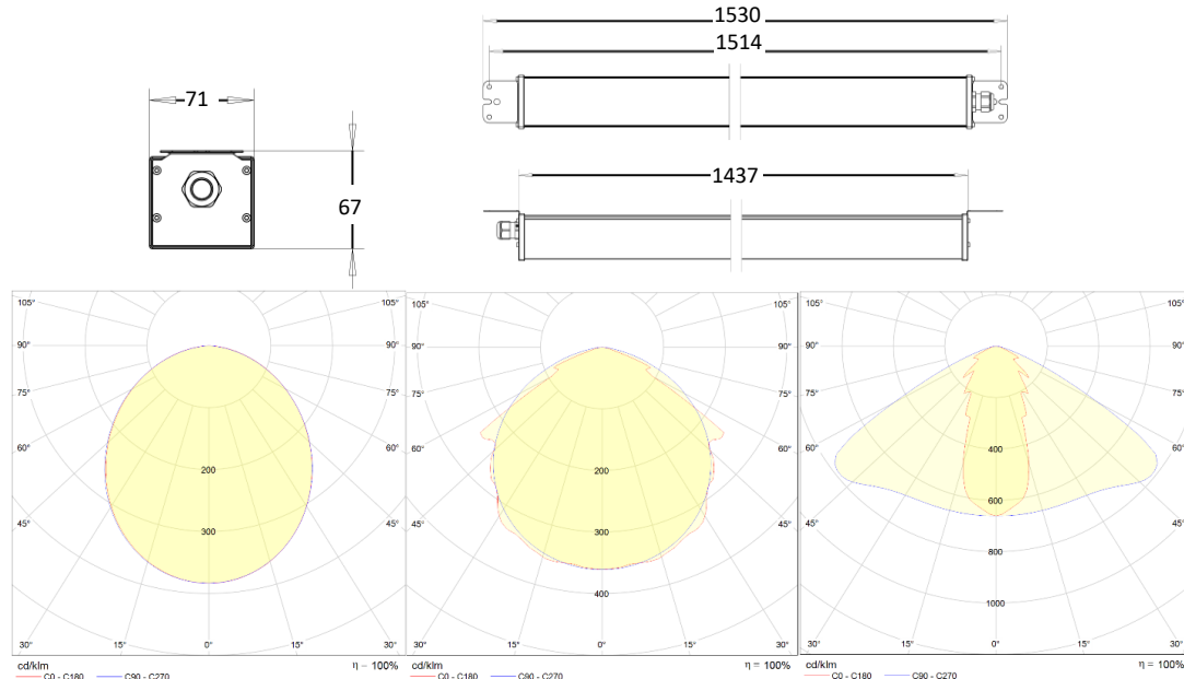
Opaalikuvun valonjako
