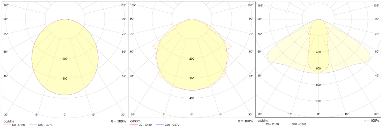
Opaalikuvun valonjako
